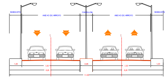
SECCION TIPO 1 - 1' PROYECTO ESC: 1/10
