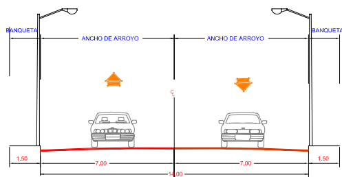
SECCION TIPO 1 - 1' PROYECTO ESC: 3/8"
